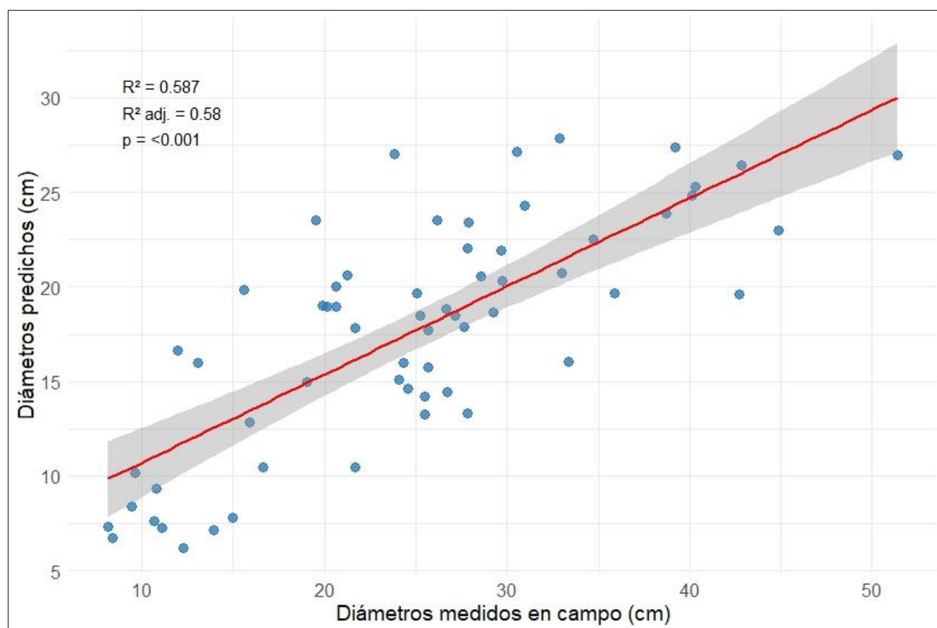
Figura 5. Relación de diámetros estimados con VANT vs diámetros medidos en campo. Figure 5. Relationship of diameters estimated with UAV vs diameters measured in the field
